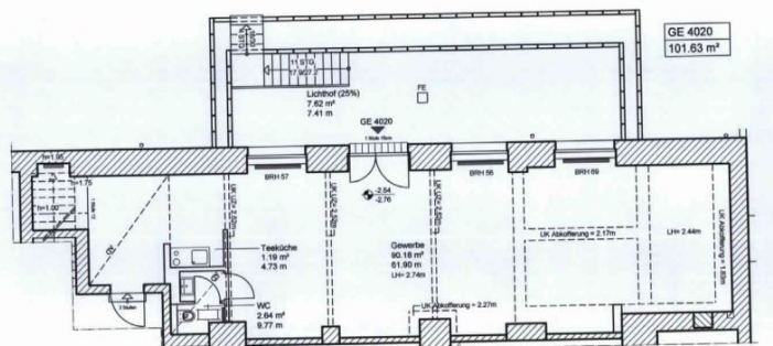
Grundriss
