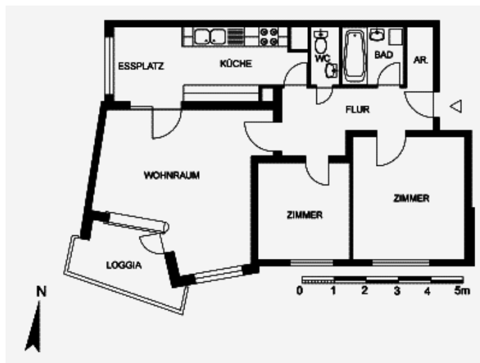
Grundriss
