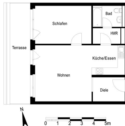
Grundriss (ohne Gewähr)
